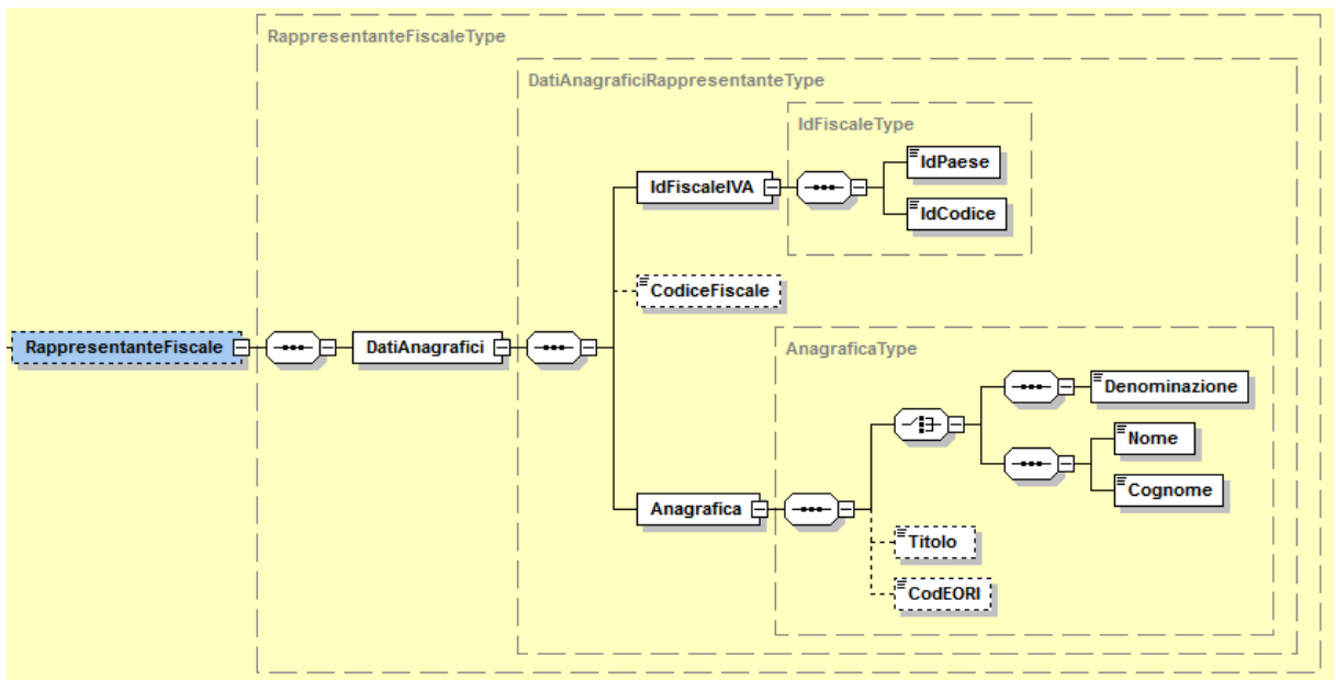
Figura 11: Elemento RappresentanteFiscale
