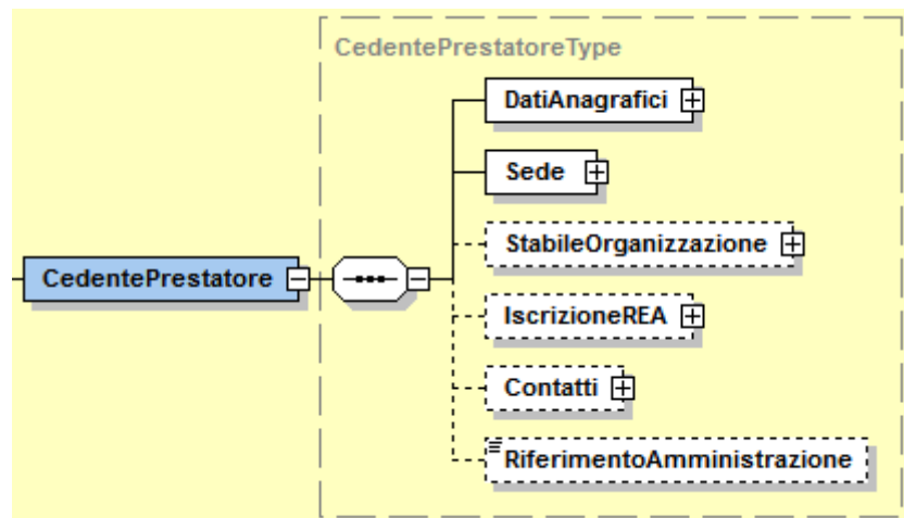
Figura 3: Elemento CedentePrestatore
