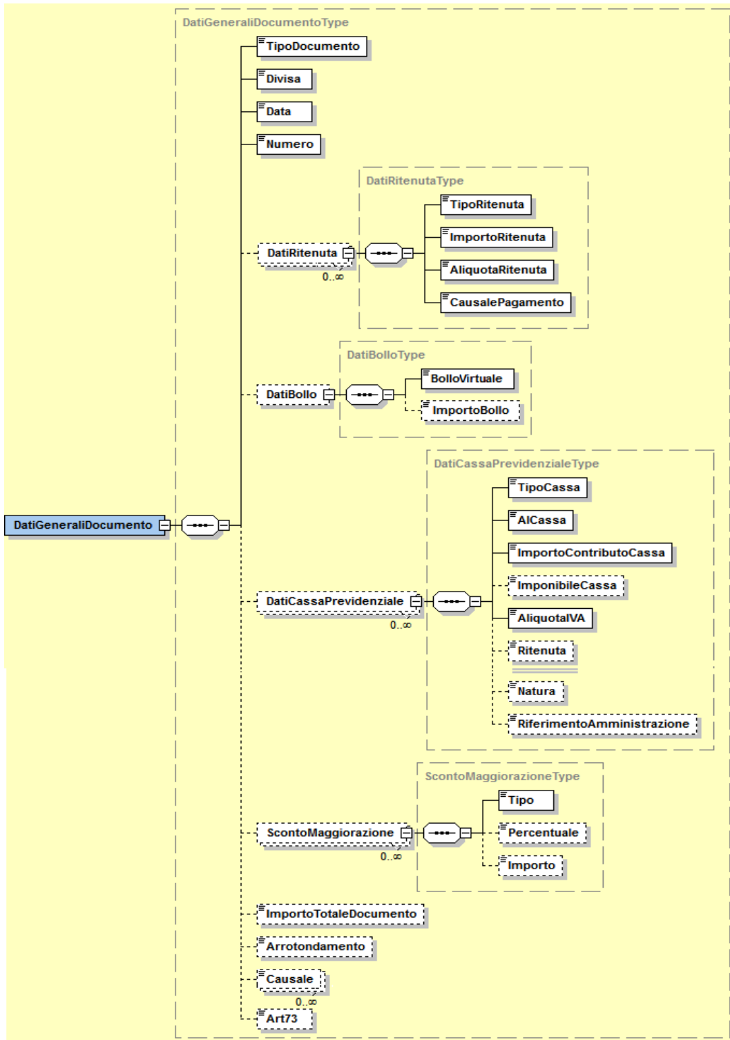
Figura 19: Elemento DatiGeneraliDocumento
